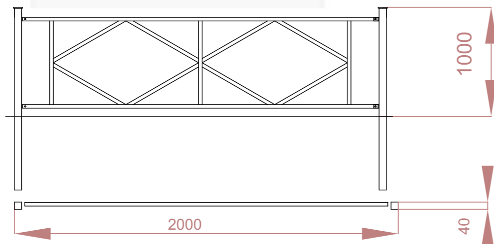
Ограда из профилтрванных труб без цоколя по металическим столбам
